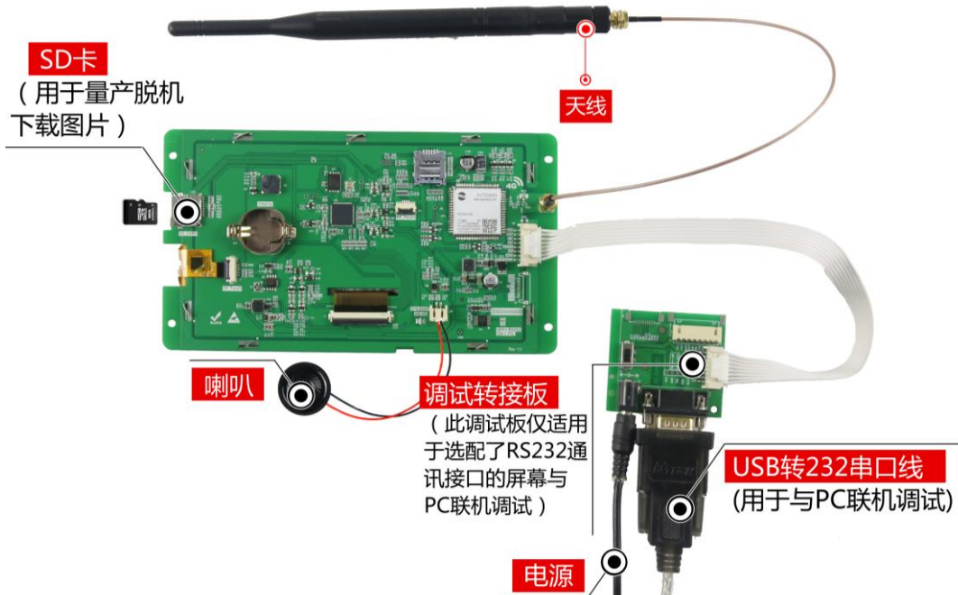
图 1-5 调试工具图
