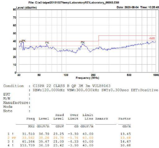
图 4-6 RE 测试垂直方向
