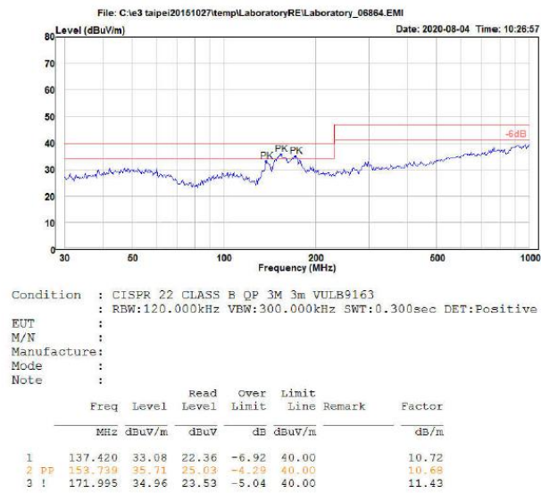
图 4-5 RE 测试水平方向
