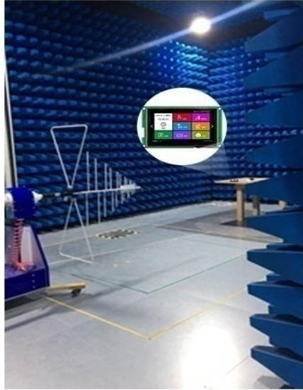
图 4-4 RE 测试图
