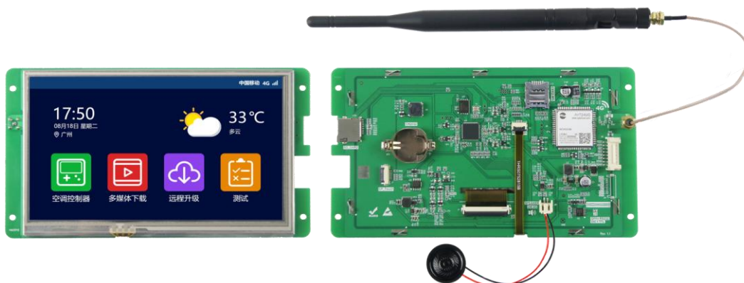
图 1-1 7.0 寸电阻触摸参考图
