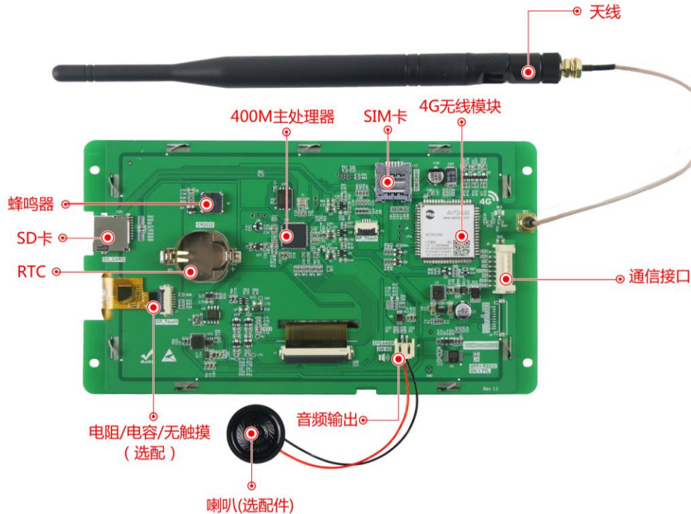
图 1-4 硬件配置图
