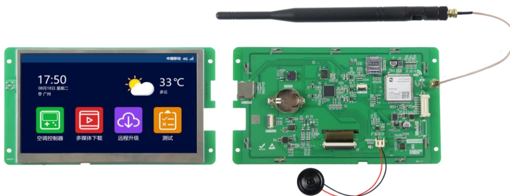
图 1-3 7.0 寸无触摸参考图
